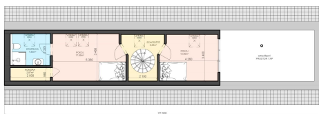
PŮDORYS PODKROVÍ
