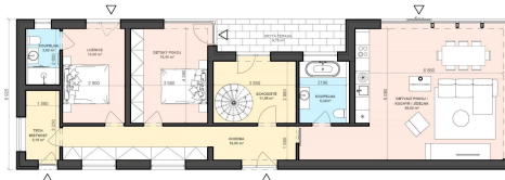
PŮDORYS PŘÍZEMÍ
