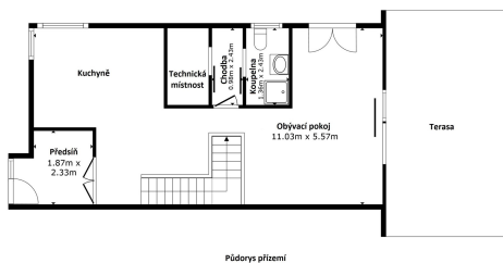
Půdorys přízemí
