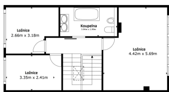
Půdorys 1. patra
