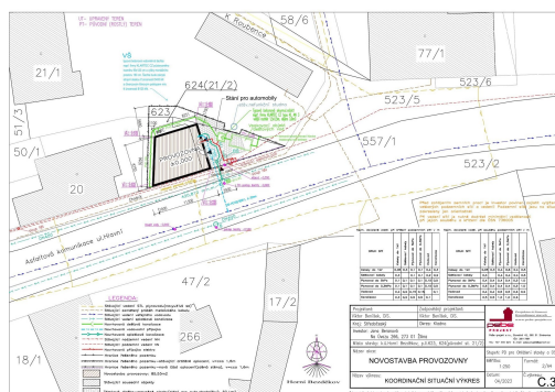
SITUACNÍ VÝKRES (1:250)
