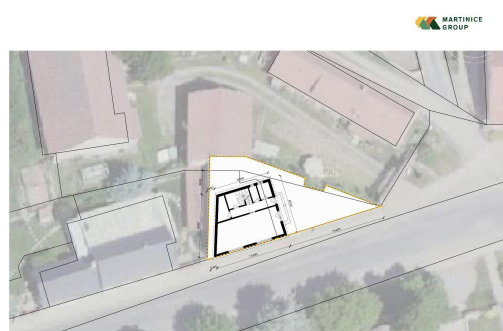
SITUACNÍ VÝKRES (1:250)
