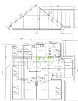
BYT POKROVÍ MOSKEVSKÁ UL , MĚŘ: 1:100
