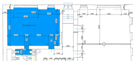
STELNÍ 123, Kaplice Legenda PŘÍZEMÍ
