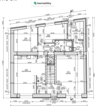
PŮDORYS 1NP
