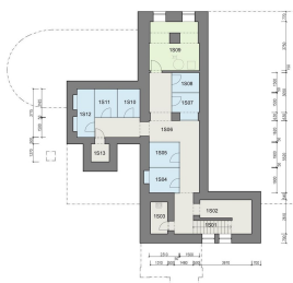
PŮDORYS SUTERÉNU
