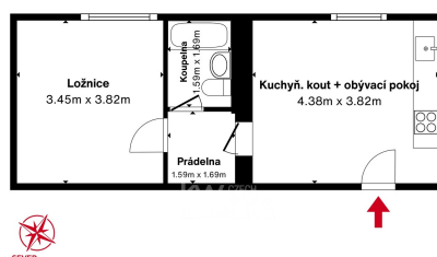
PŮDORYS
