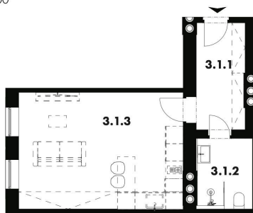
PŮDORYS BYTU 1:100
