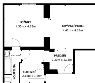
Půdorys suterénu
