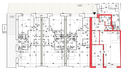
PŮDORYS 1.NP
