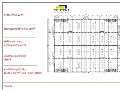
Půdorys
